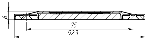
СЕЧЕНИЕ А-А
